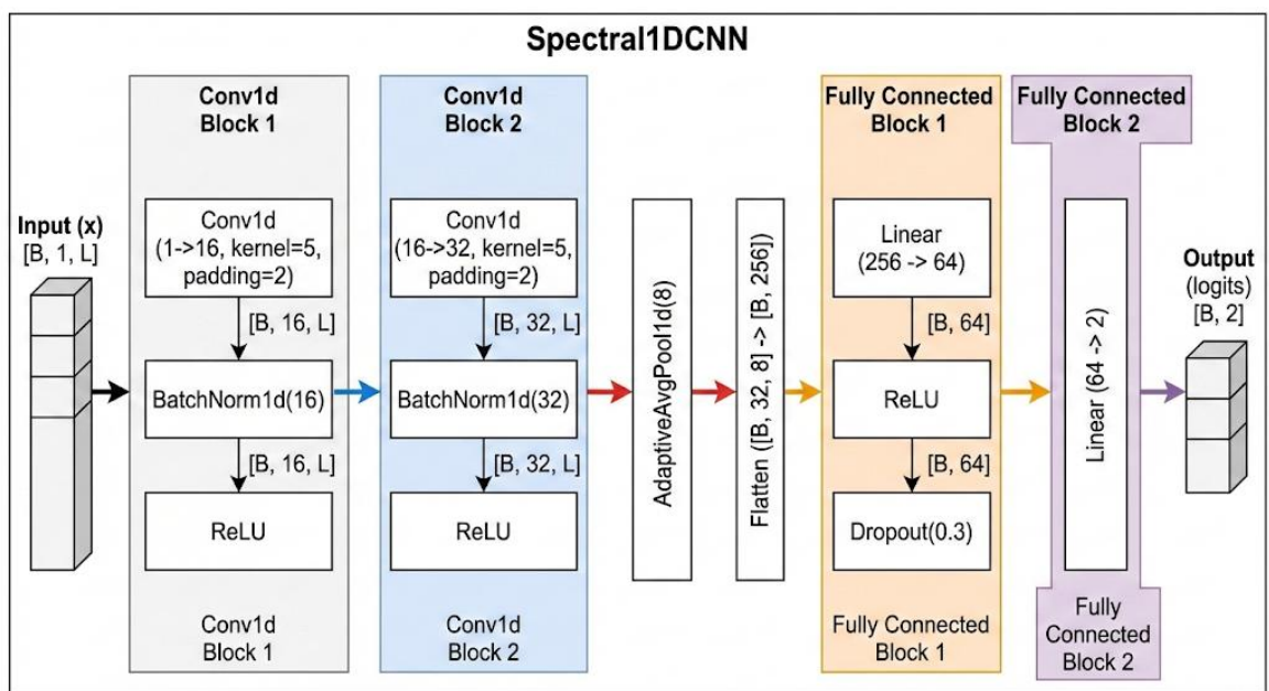
Figura 3-5: Arquitectura propuesta para la CNN-1D con parámetros default. Las arquitecturas fueron esquematizadas a partir de la implementación en PyTorch. Los valores de canales y dimensiones corresponden a la configuración utilizada en este estudio
